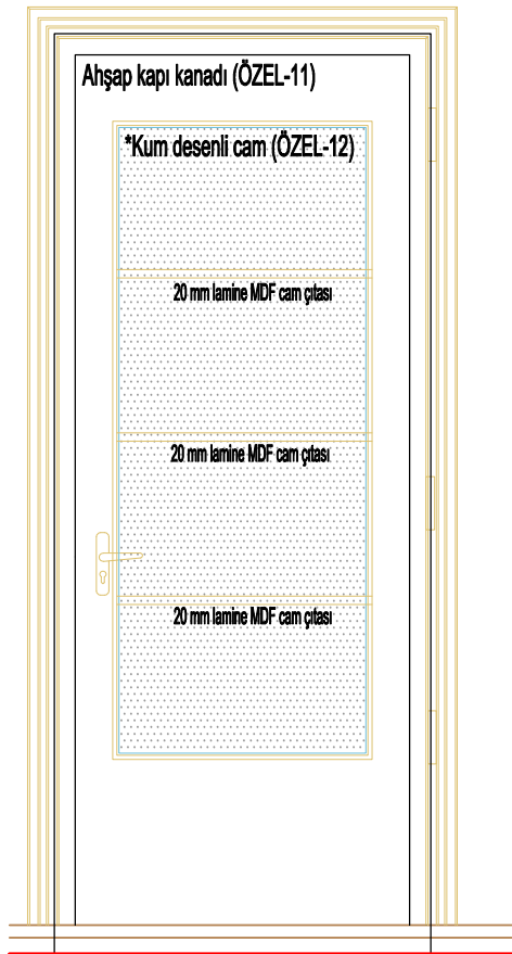
GÖRÜNÜŞ Ö:1/20
