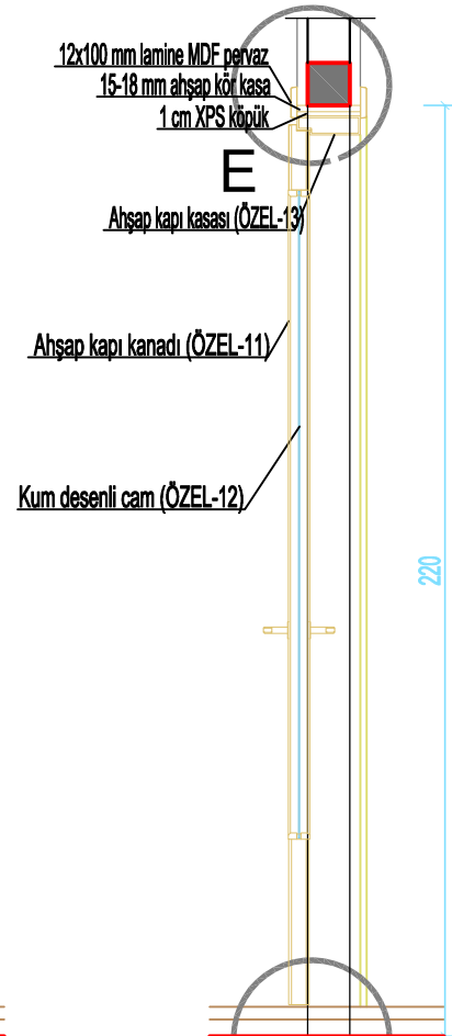
KESİT Ö:1/20
